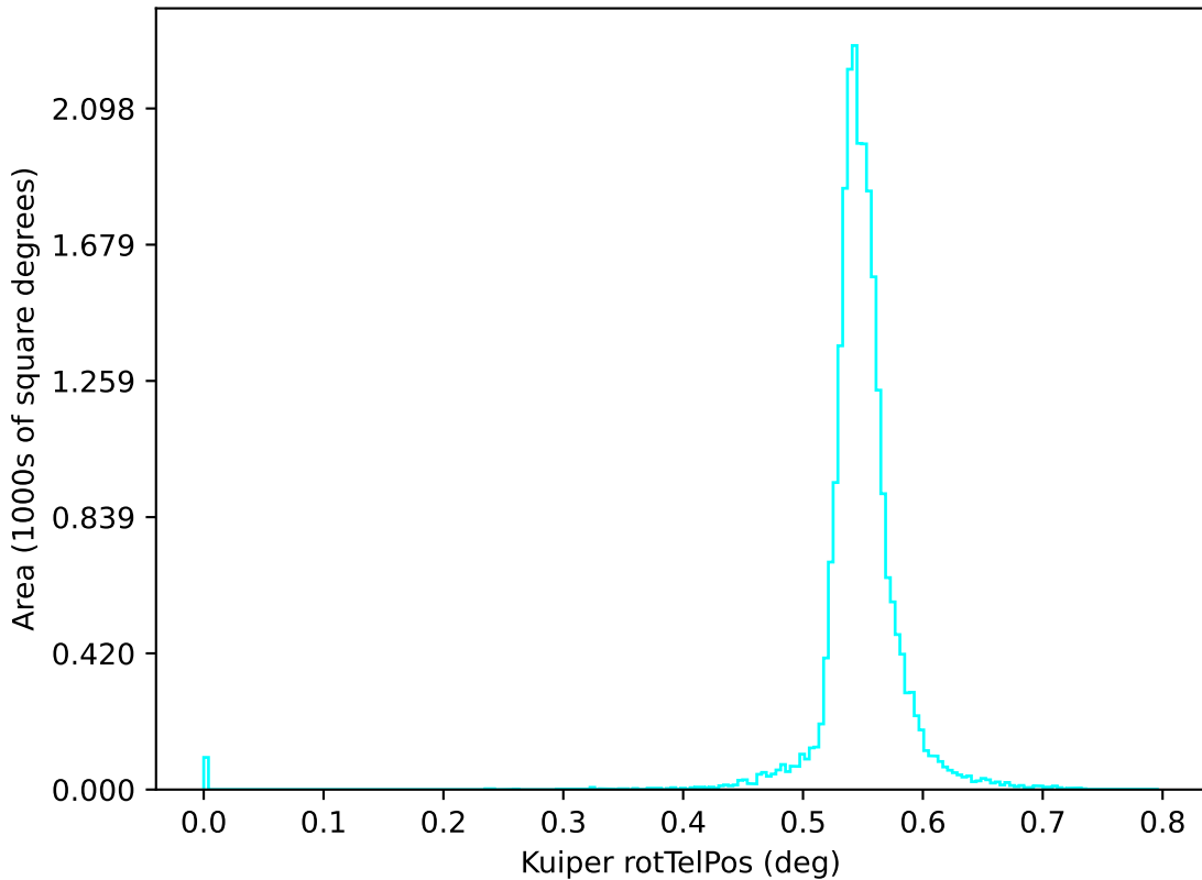
ddf_acor_sf10_lsf20_lsr10_v3.4_10yrs u: Kuiper rotTelPos
