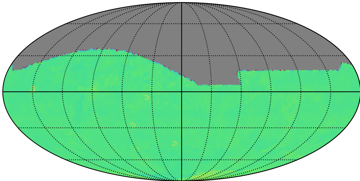
ddf_acor_sf10_lsf20_lsr10_v3.4_10yrs r: Kuiper rotTelPos
