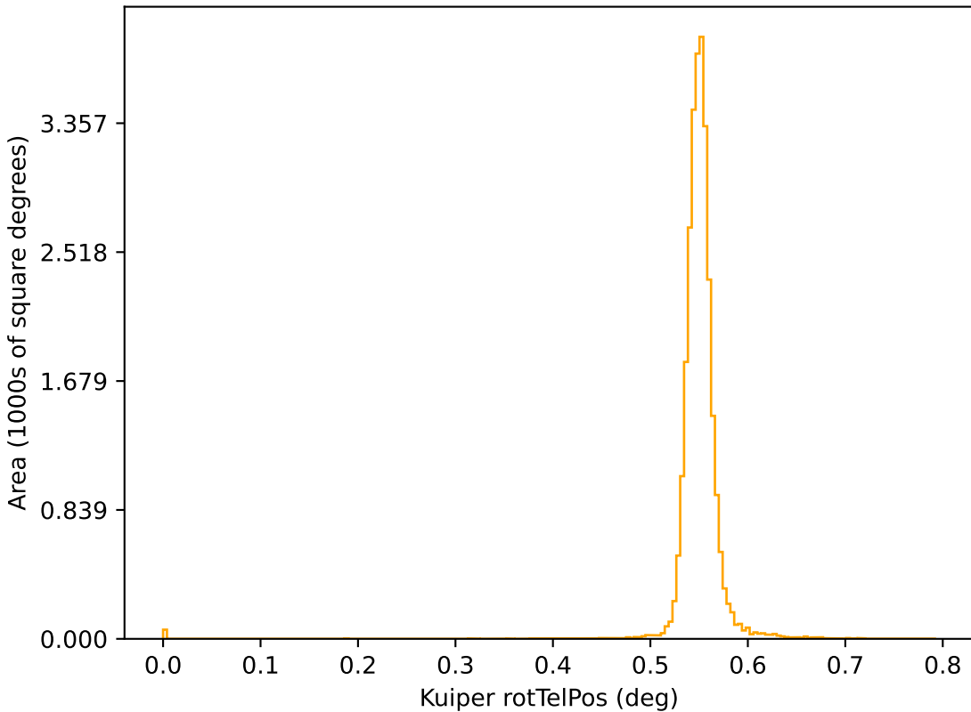
ddf_acor_sf10_lsf20_lsr10_v3.4_10yrs r: Kuiper rotTelPos
