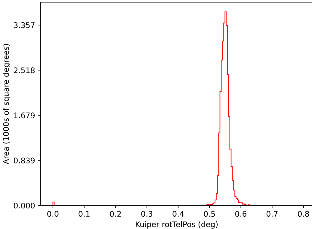
ddf_acor_sf10_lsf20_lsr10_v3.4_10yrs i: Kuiper rotTelPos
