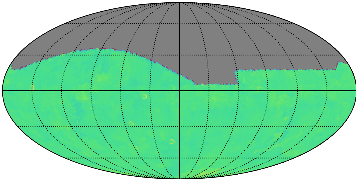
ddf_acor_sf10_lsf20_lsr10_v3.4_10yrs g: Kuiper rotTelPos
