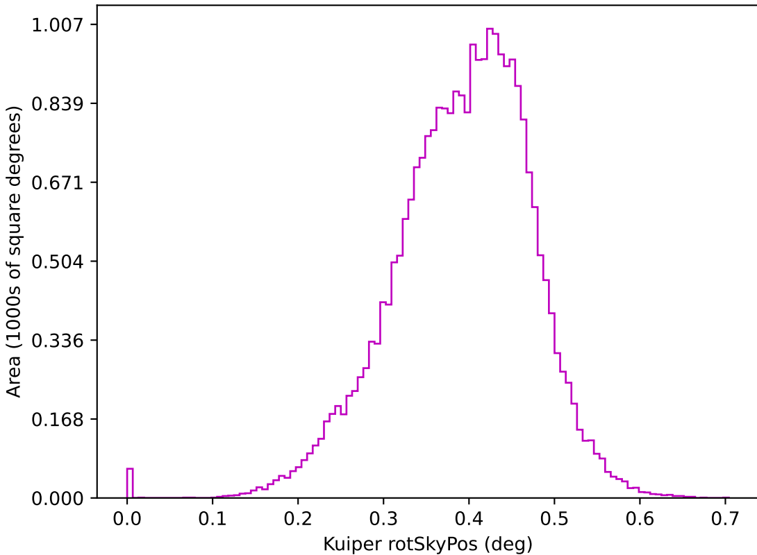
ddf_acor_sf10_lsf20_lsr10_v3.4_10yrs z: Kuiper rotSkyPos
