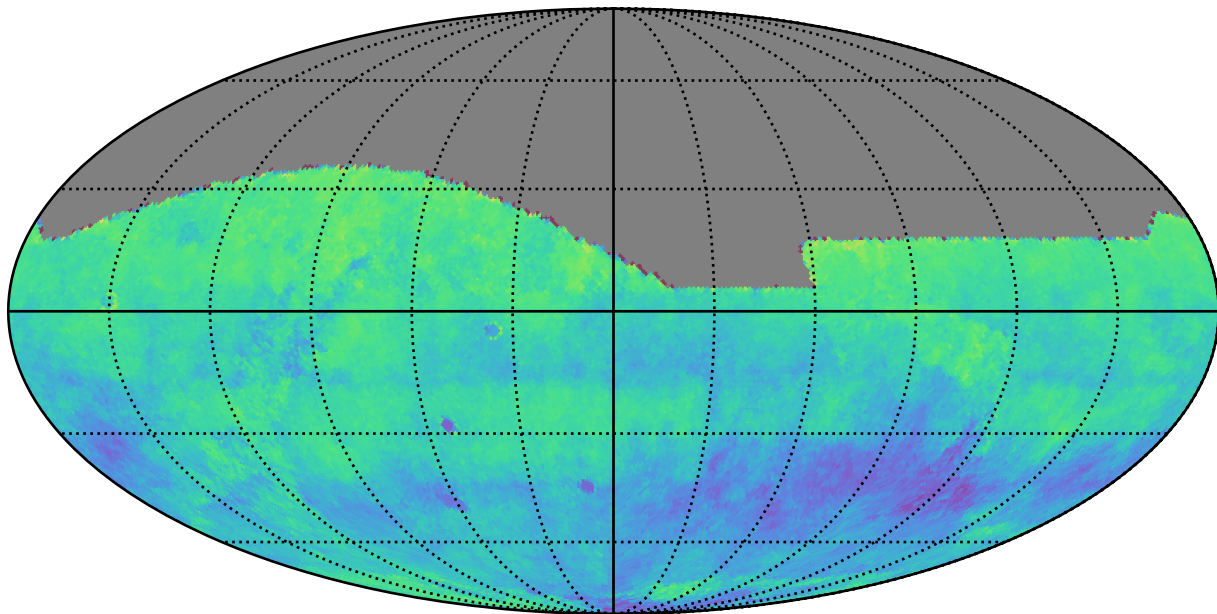
ddf_acor_sf10_lsf20_lsr10_v3.4_10yrs i: Kuiper rotSkyPos
