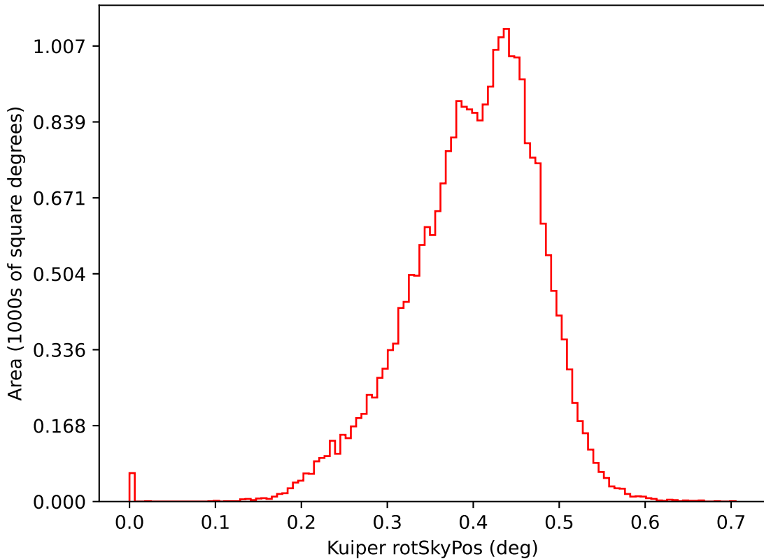
ddf_acor_sf10_lsf20_lsr10_v3.4_10yrs i: Kuiper rotSkyPos
