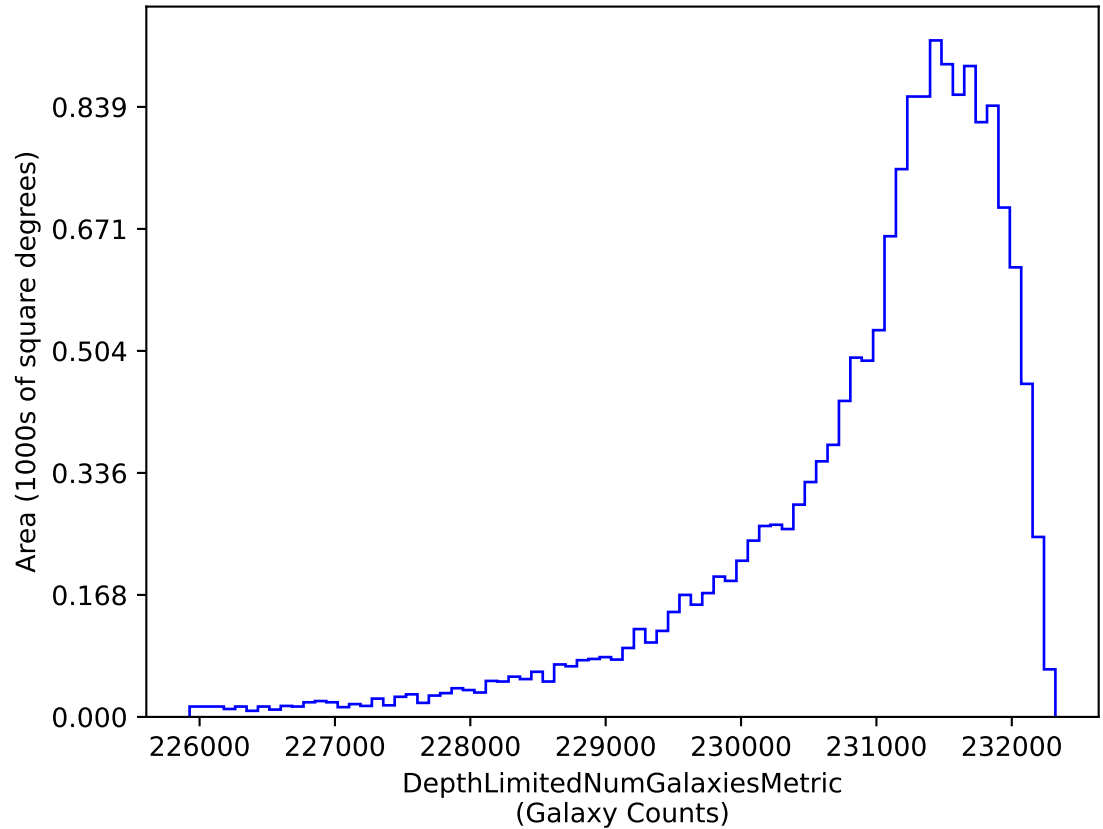
ddf_acor_sf10_lsf20_lsr10_v3.4_10yrs i band galaxies non-DD: DepthLimitedNumGalaxiesMetric
