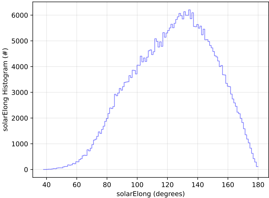
ddf_acor_sf10_lsf20_lsr10_v3.4_10yrs All sky y band: solarElong Histogram
