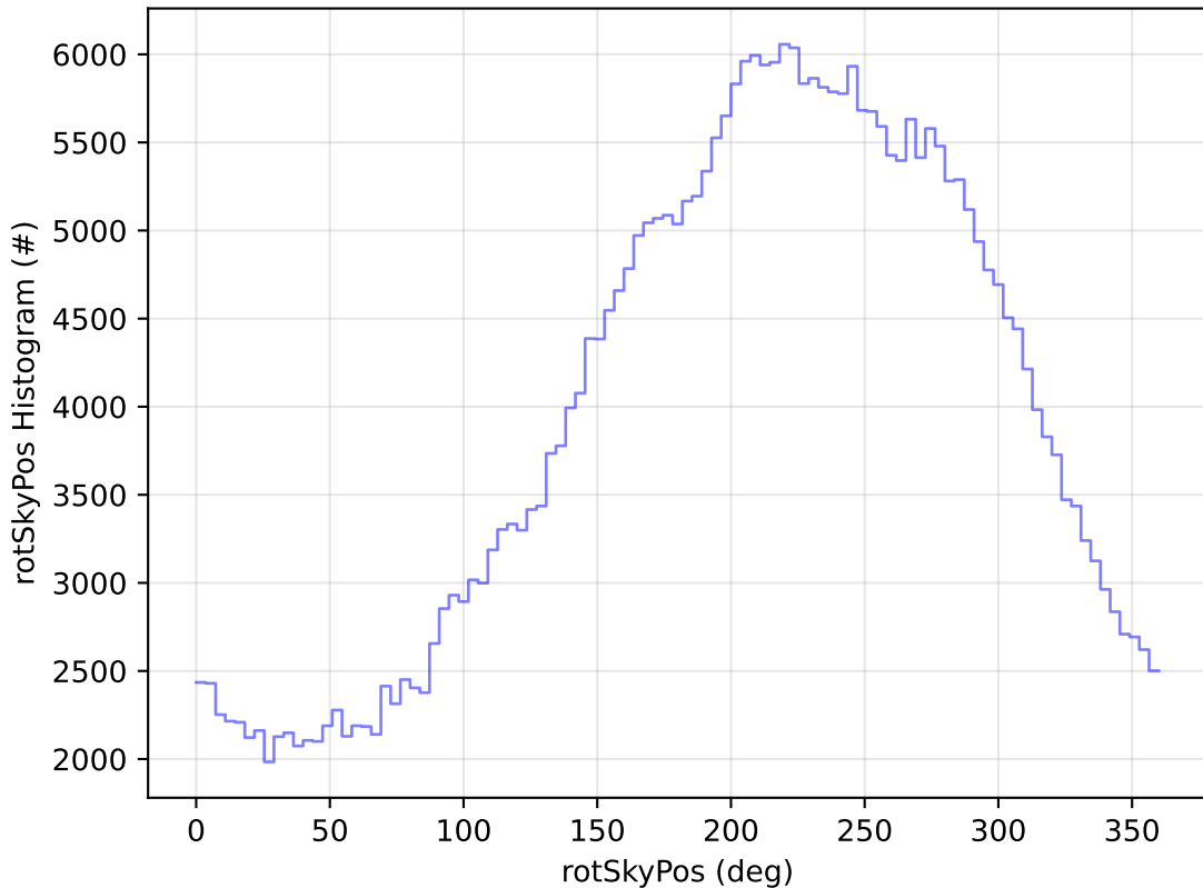
ddf_acor_sf10_lsf20_lsr10_v3.4_10yrs WFD y band: rotSkyPos Histogram
