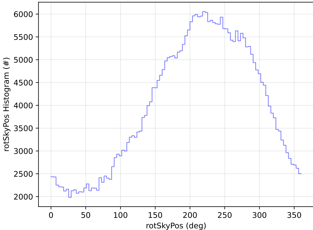
ddf_acor_sf10_lsf20_lsr10_v3.4_10yrs All sky y band: rotSkyPos Histogram
