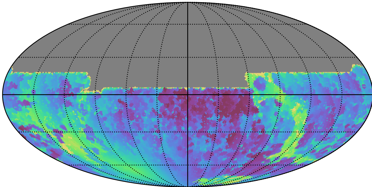
ddf_acor_sf10_lsf20_lsr10_v3.4_10yrs All sky y band: Min solarElong
