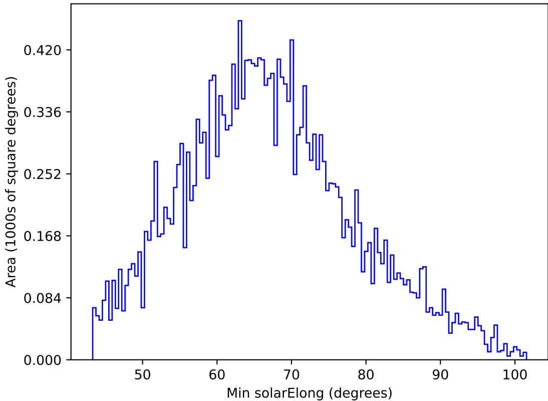
ddf_acor_sf10_lsf20_lsr10_v3.4_10yrs All sky y band: Min solarElong
