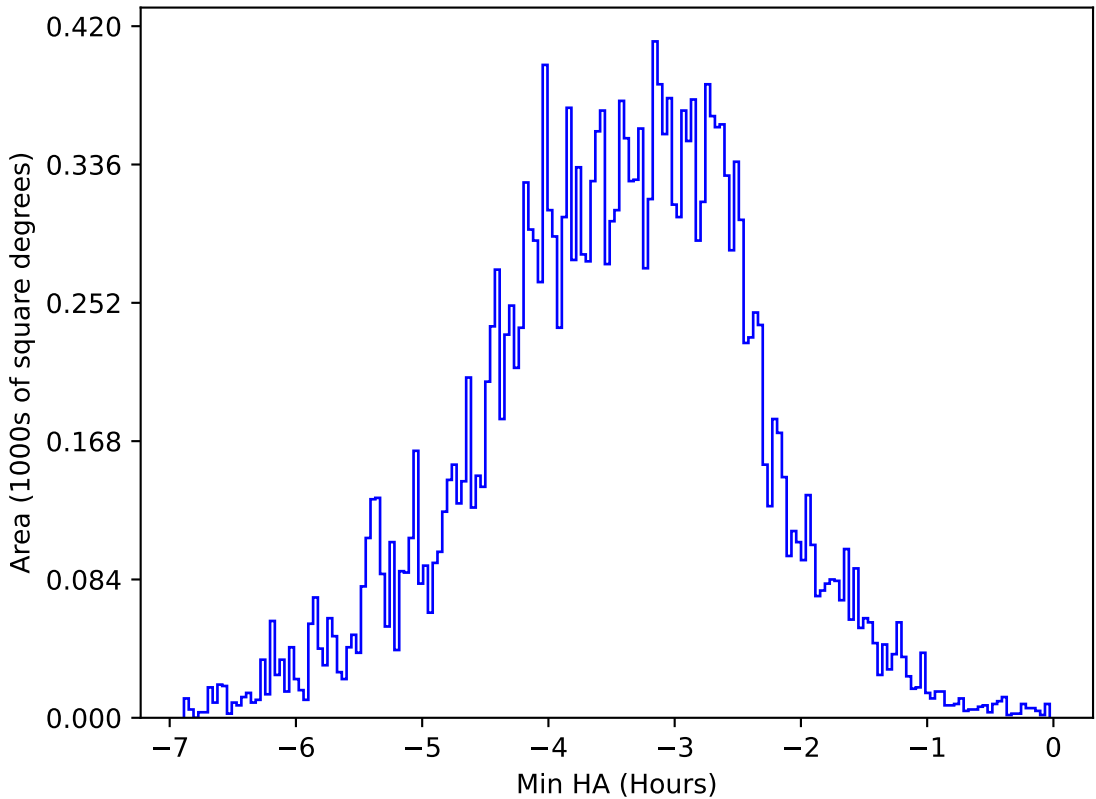
ddf_acor_sf10_lsf20_lsr10_v3.4_10yrs All sky y band: Min HA
