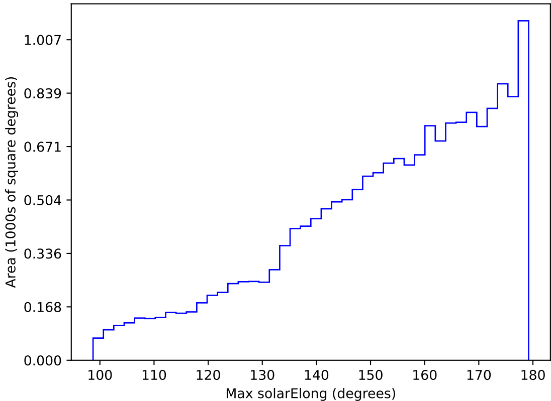
ddf_acor_sf10_lsf20_lsr10_v3.4_10yrs WFD y band: Max solarElong
