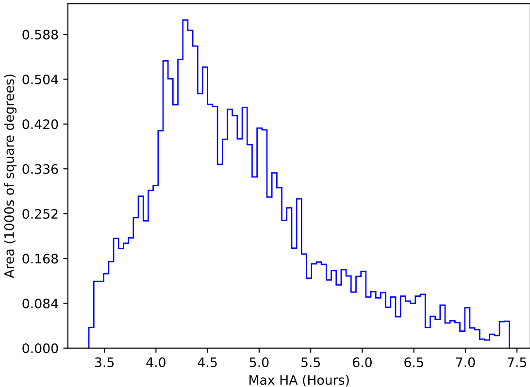
ddf_acor_sf10_lsf20_lsr10_v3.4_10yrs WFD y band: Max HA
