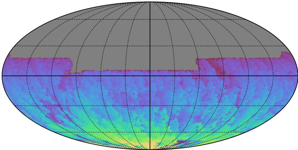
ddf_acor_sf10_lsf20_lsr10_v3.4_10yrs All sky y band: Max HA
