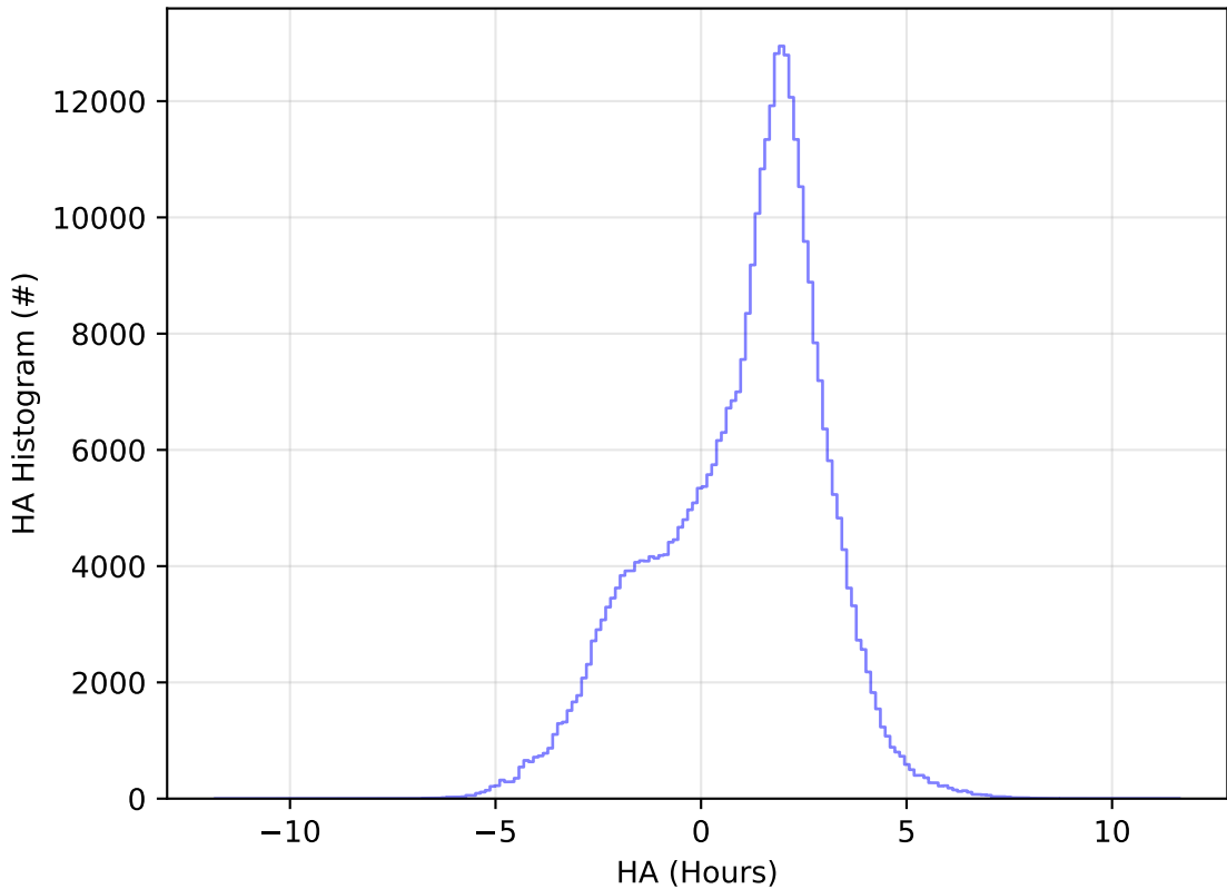
ddf_acor_sf10_lsf20_lsr10_v3.4_10yrs All sky y band: HA Histogram
