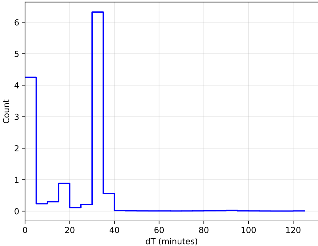
ddf_acor_sf10_lsf20_lsr10_v3.4_10yrs All sky: DeltaT Histogram 1e6
