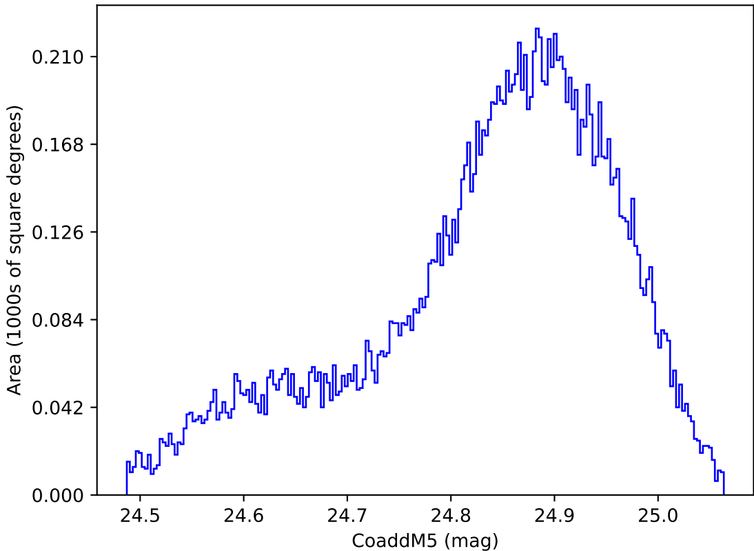
ddf_acor_sf10_lsf20_lsr10_v3.4_10yrs WFD y band: CoaddM5
