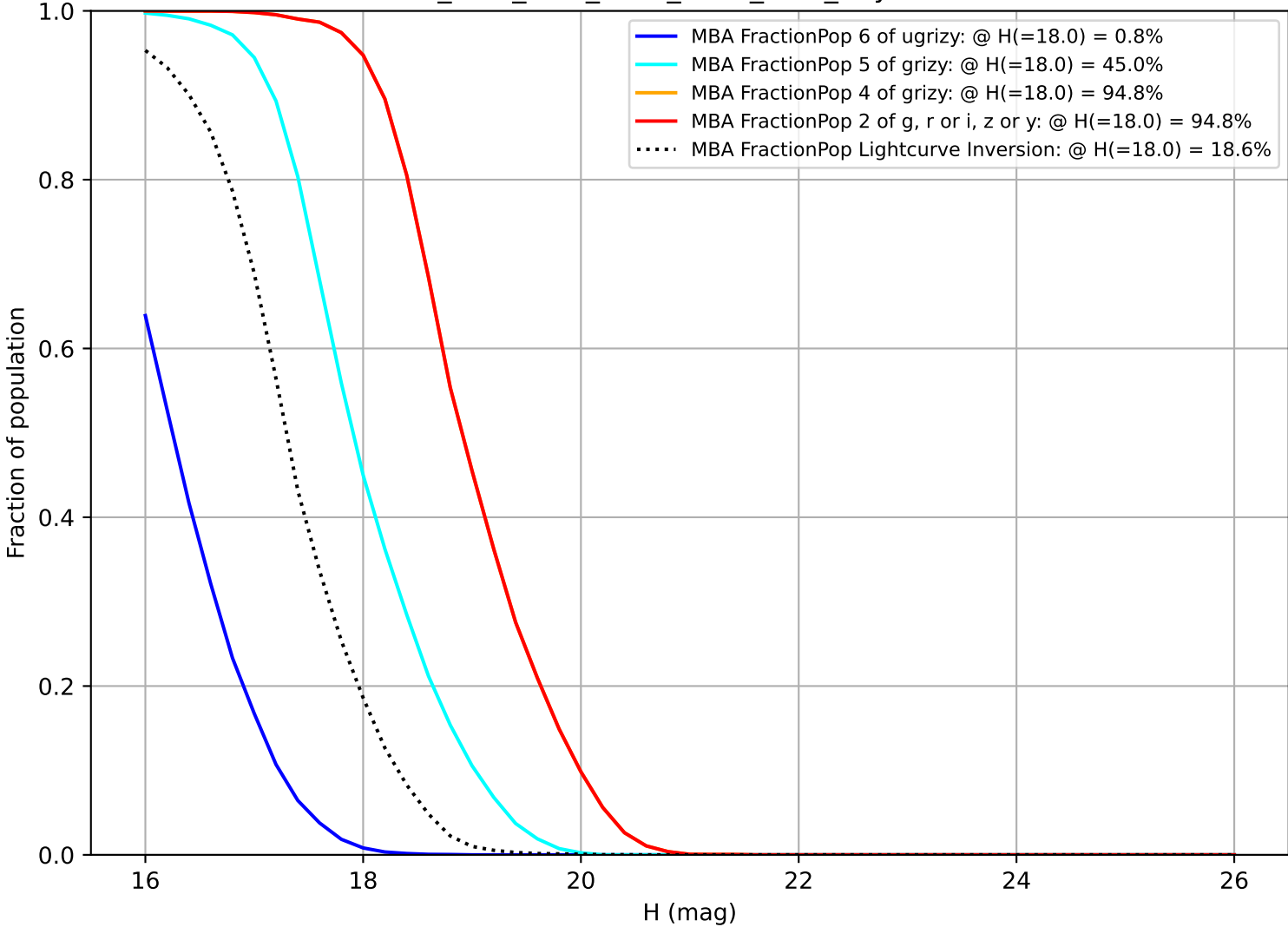
ddf_acor_sf10_lsf15_lsr50_v3.4_10yrs MBA
