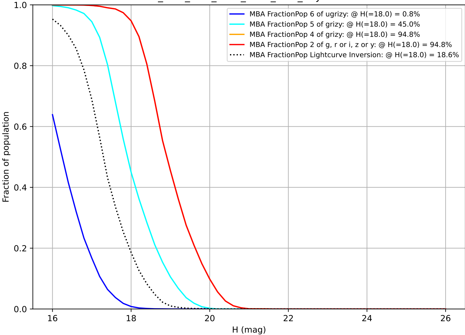
ddf_acor_sf10_lsf15_lsr50_v3.4_10yrs MBA
