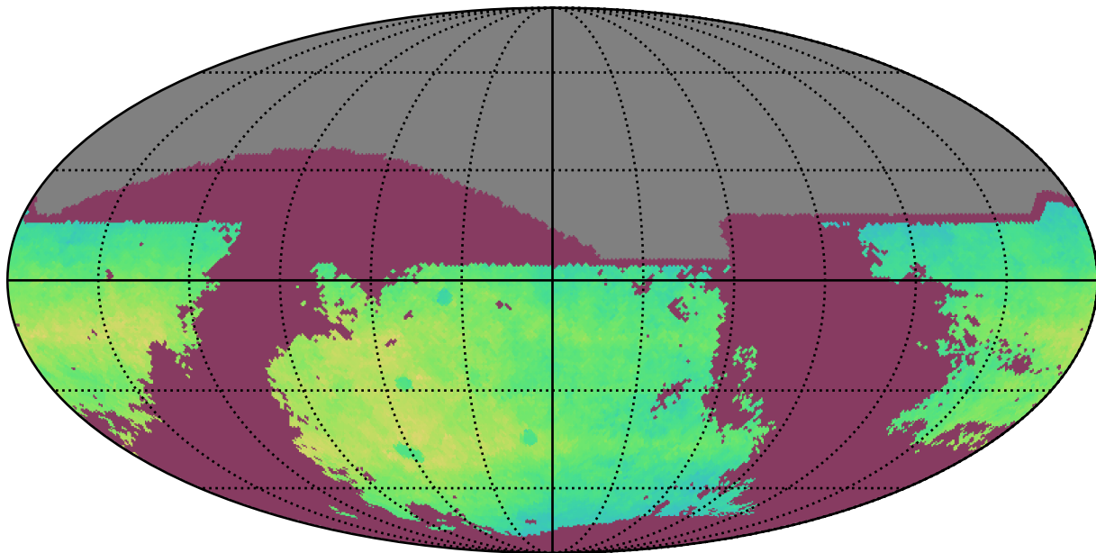
ddf_acor_sf10_lsf15_lsr50_v3.4_10yrs i: NgalScale
