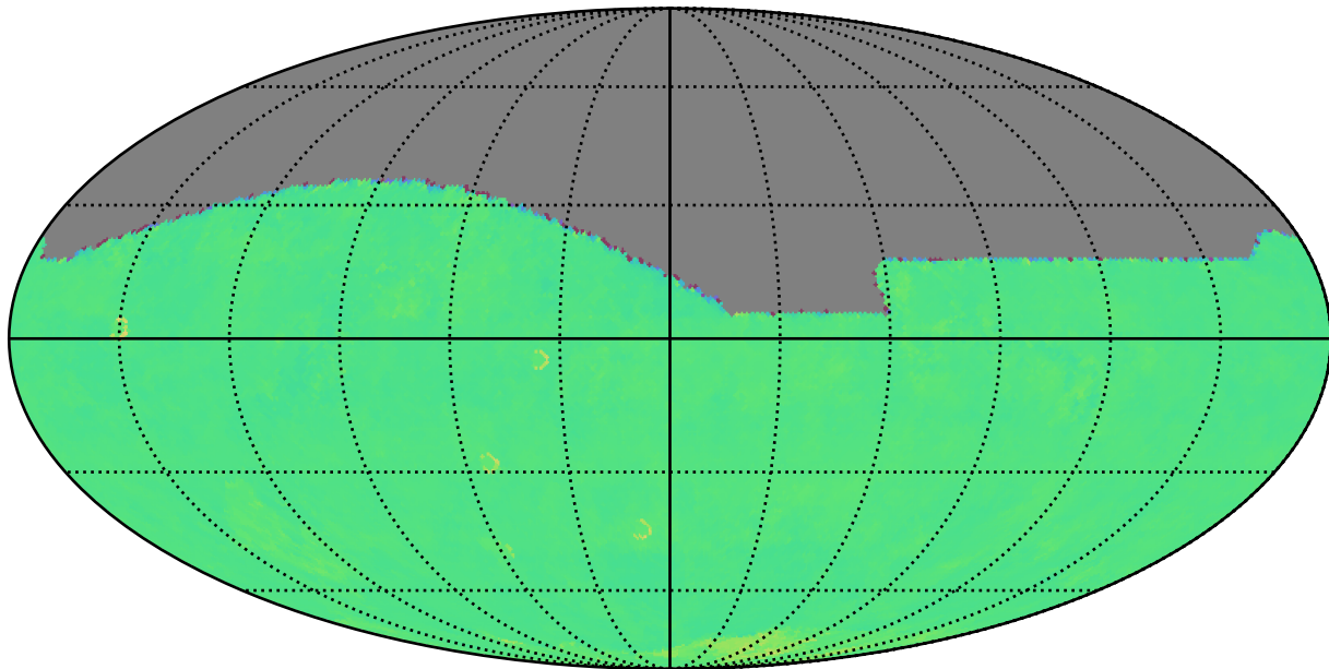
ddf_acor_sf10_lsf15_lsr50_v3.4_10yrs r: Kuiper rotTelPos
