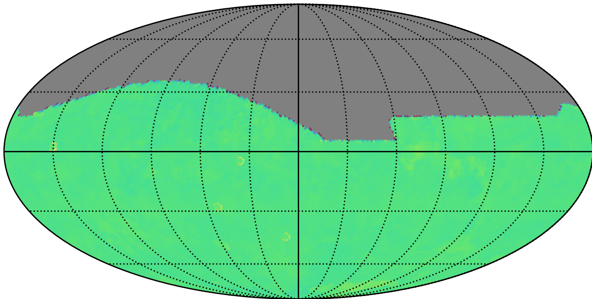
ddf_acor_sf10_lsf15_lsr50_v3.4_10yrs i: Kuiper rotTelPos
