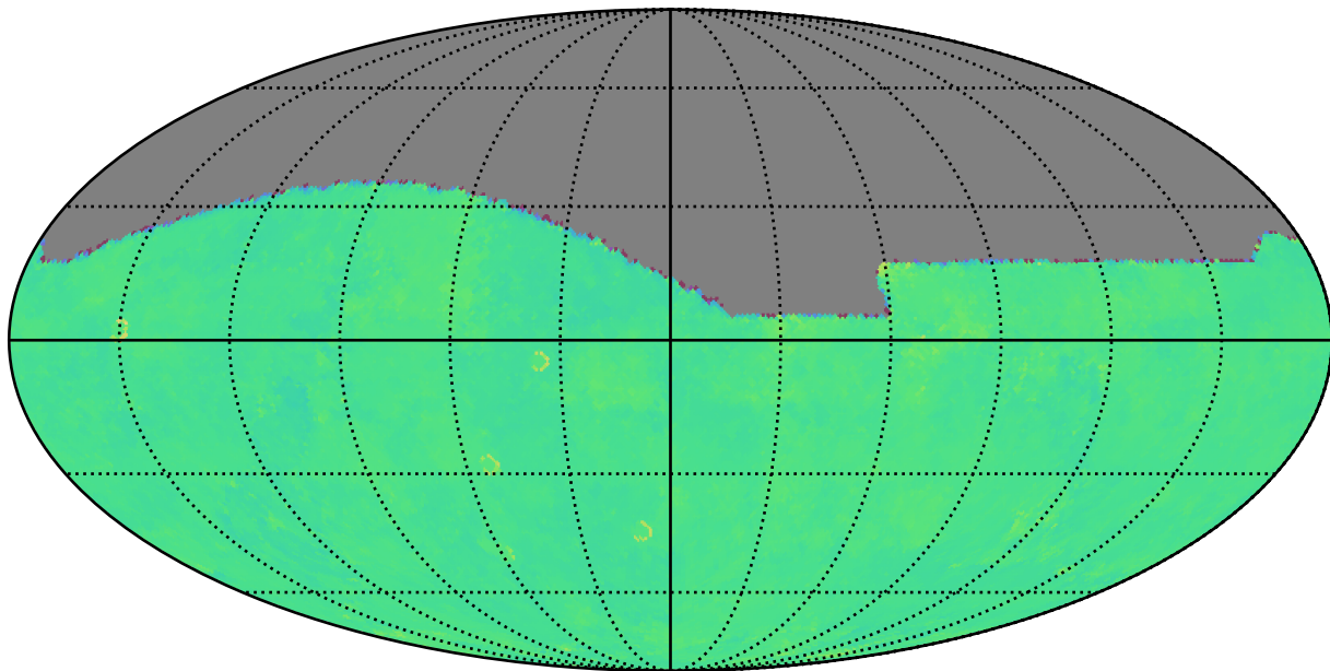
ddf_acor_sf10_lsf15_lsr50_v3.4_10yrs g: Kuiper rotTelPos
