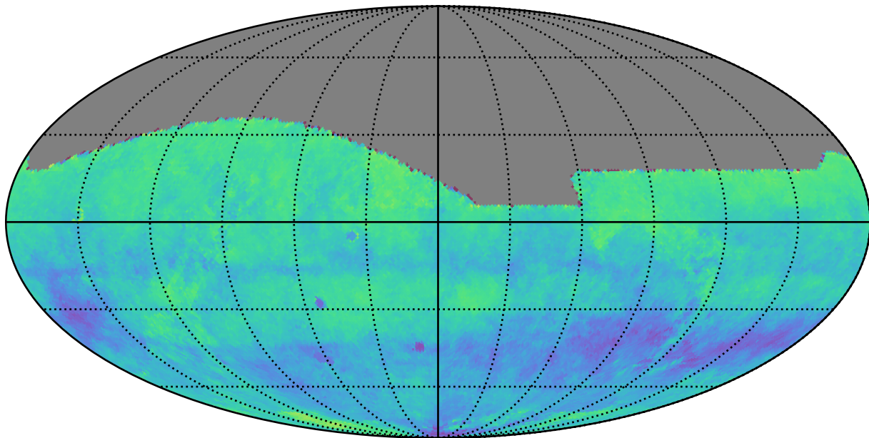
ddf_acor_sf10_lsf15_lsr50_v3.4_10yrs i: Kuiper rotSkyPos
