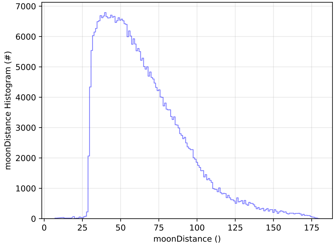
ddf_acor_sf10_lsf15_lsr50_v3.4_10yrs All sky y band: moonDistance Histogram
