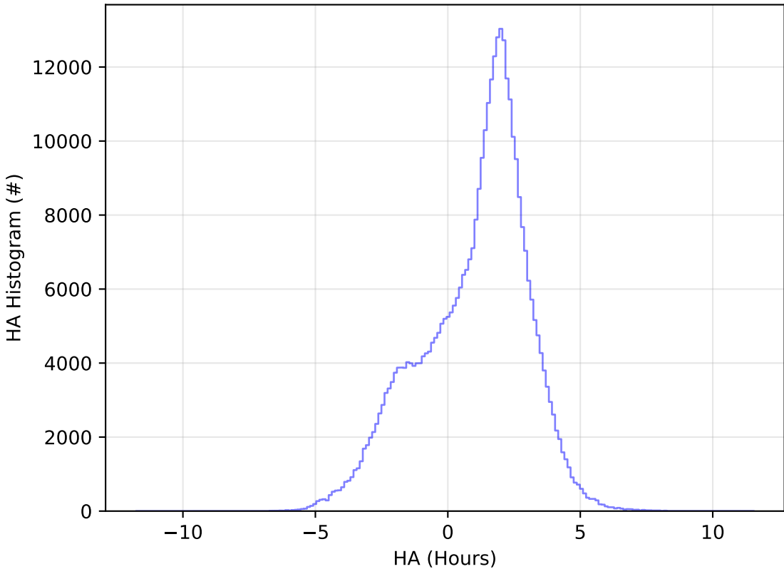
ddf_acor_sf10_lsf15_lsr50_v3.4_10yrs WFD y band: HA Histogram
