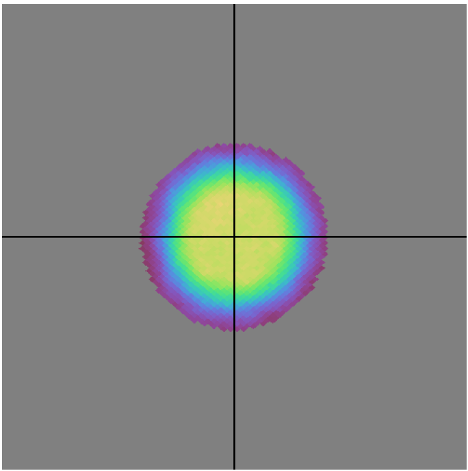
ddf_acor_sf10_lsf15_lsr50_v3.4_10yrs all bands: DD:COSMOS N Unique Nights
