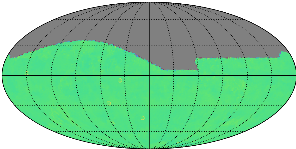
ddf_acor_sf10_lsf15_lsr20_v3.4_10yrs i: Kuiper rotTelPos
