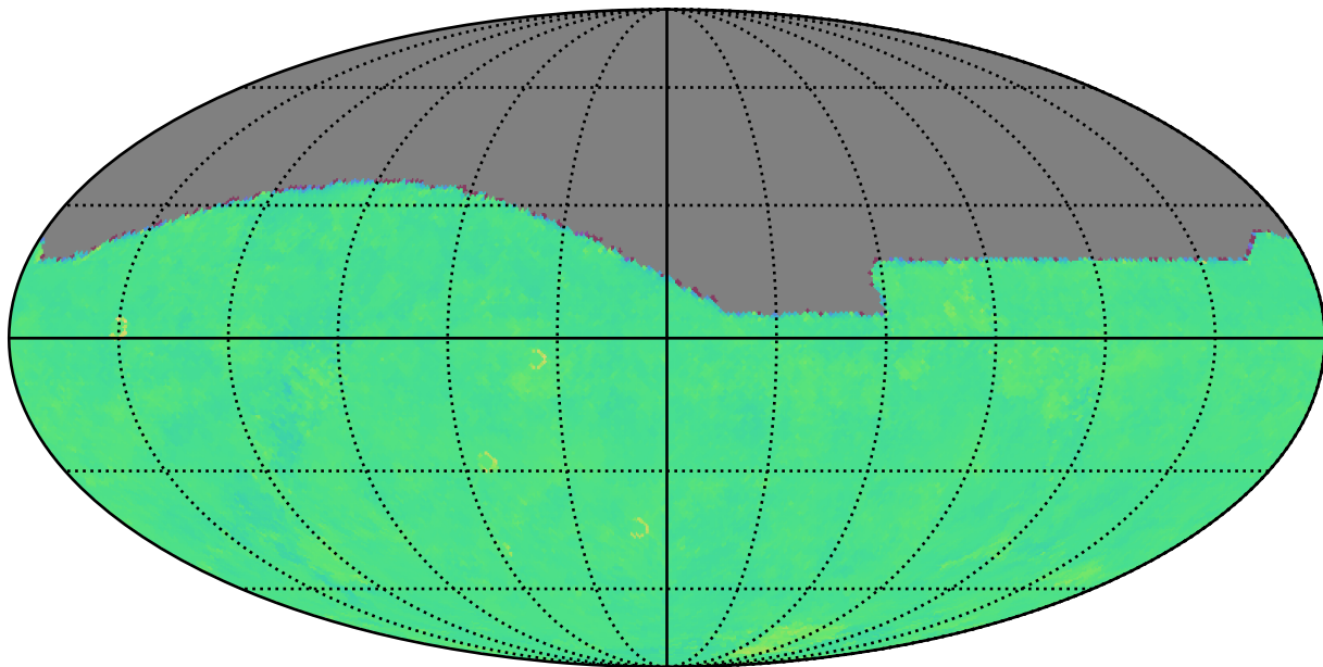
ddf_acor_sf10_lsf15_lsr20_v3.4_10yrs g: Kuiper rotTelPos
