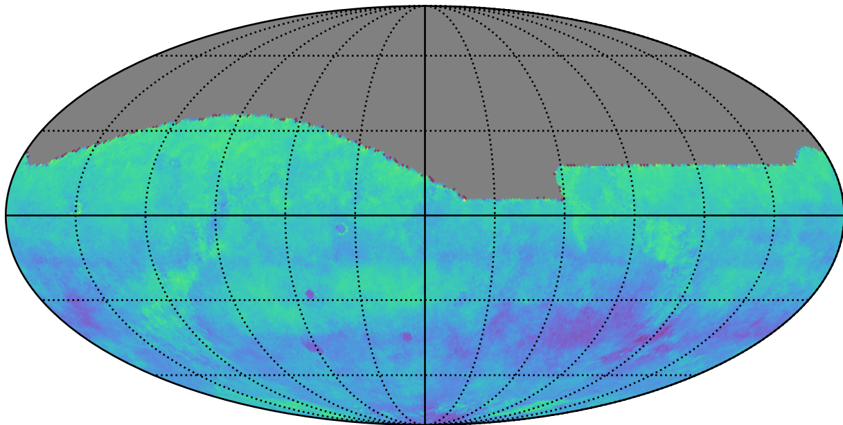
ddf_acor_sf10_lsf15_lsr20_v3.4_10yrs i: Kuiper rotSkyPos
