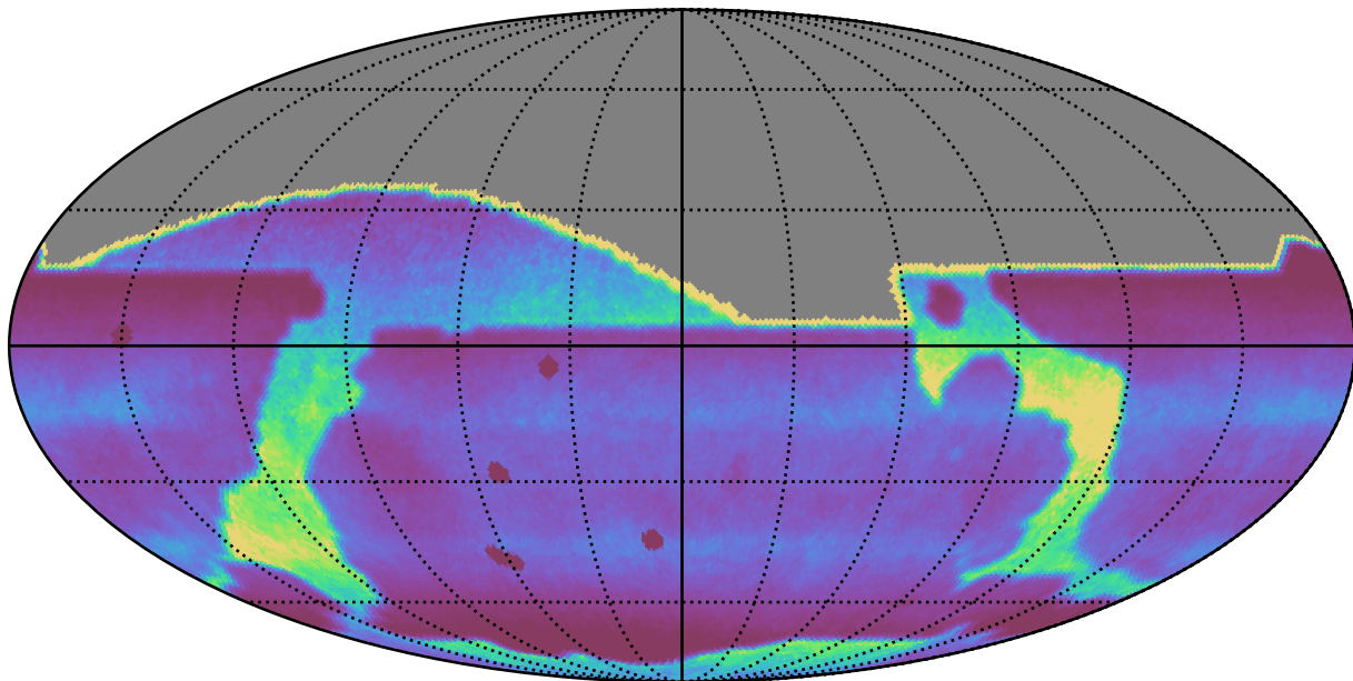
ddf_acor_sf10_lsf15_lsr20_v3.4_10yrs : DCRprecision
