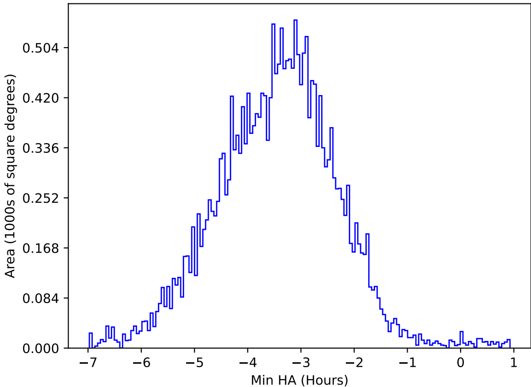
ddf_acor_sf10_ls15_lsr20_v3.4_10yrs All sky y band: Min HA
