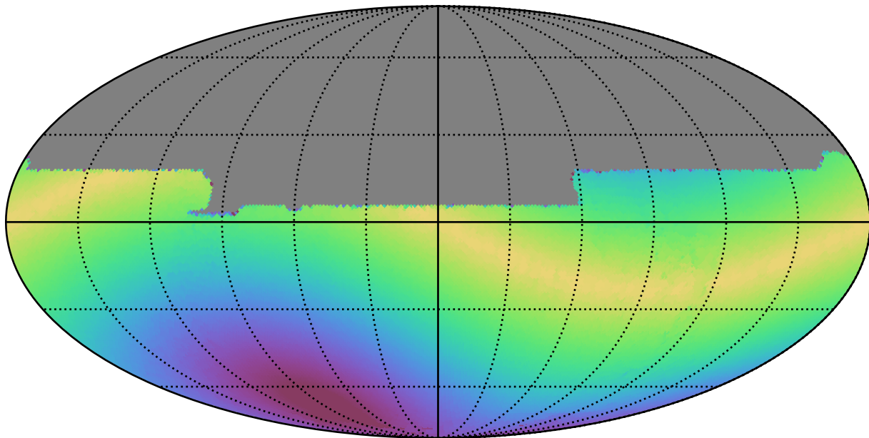
ddf_acor_sf10_lsf15_lsr20_v3.4_10yrs All sky y band: Max solarElong
