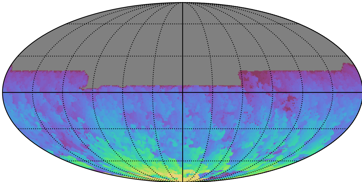
ddf_acor_sf10_lsf15_lsr20_v3.4_10yrs All sky y band: Max HA
