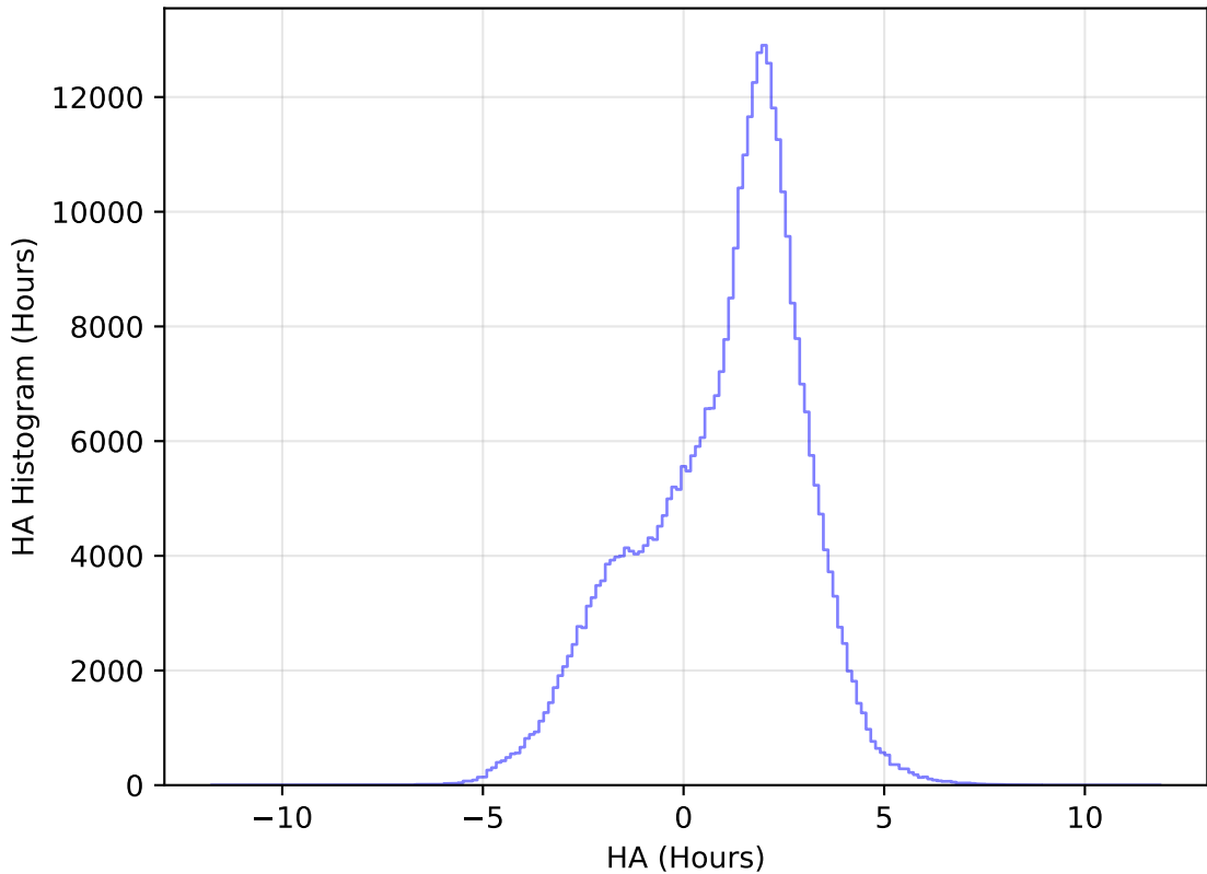
ddf_acor_sf10_lsf15_lsr20_v3.4_10yrs All sky y band: HA Histogram
