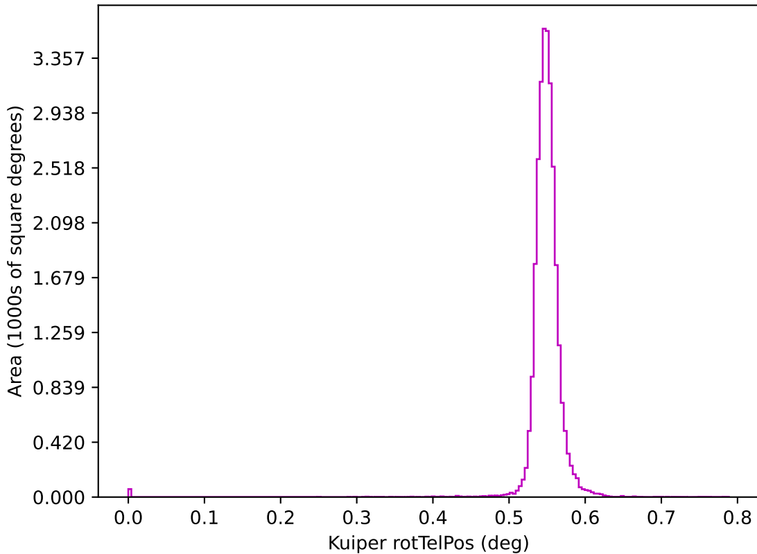
ddf_acor_sf10_lsf15_lsr10_v3.4_10yrs z: Kuiper rotTelPos
