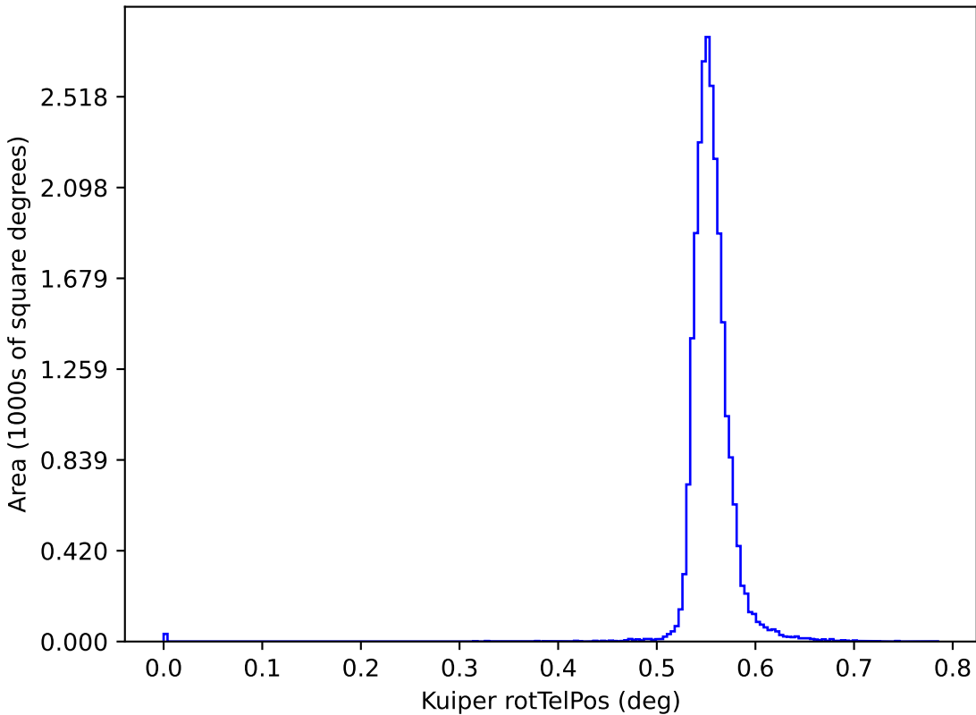
ddf_acor_sf10_lsf15_lsr10_v3.4_10yrs y: Kuiper rotTelPos
