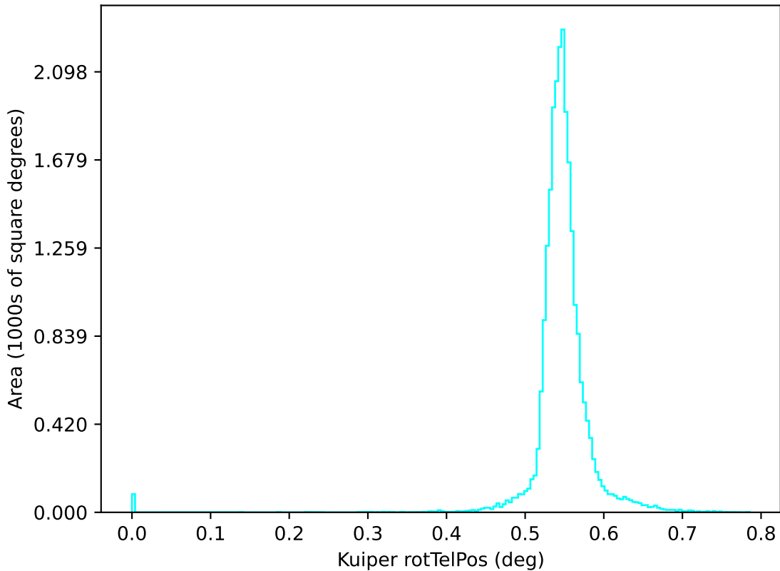
ddf_acor_sf10_ls15_lsr10_v3.4_10yrs u: Kuiper rotTelPos
