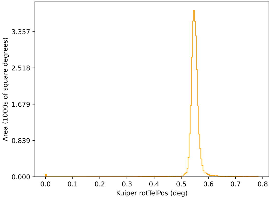
ddf_acor_sf10_lsf15_lsr10_v3.4_10yrs r: Kuiper rotTelPos
