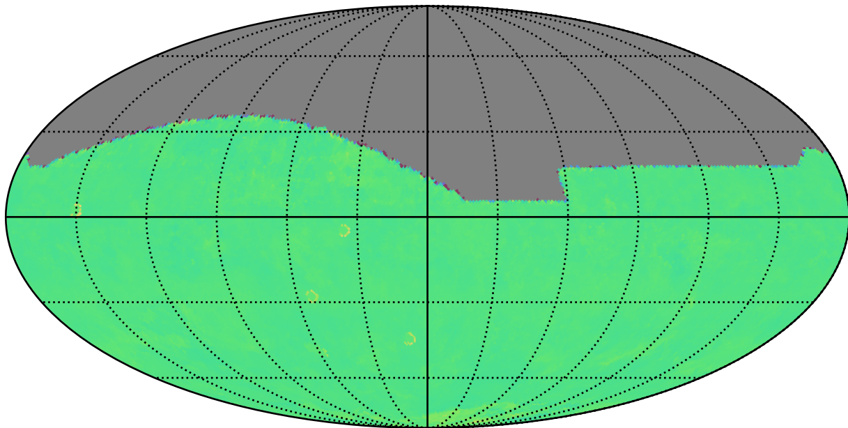
ddf_acor_sf10_lsf15_lsr10_v3.4_10yrs i: Kuiper rotTelPos
