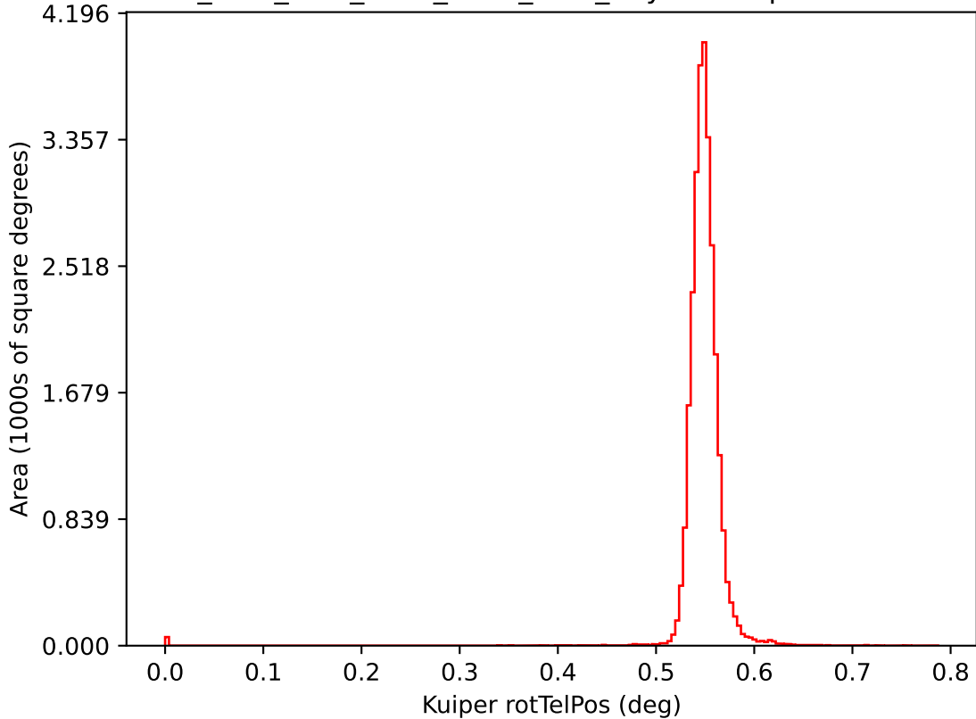
ddf_acor_sf10_lsf15_lsr10_v3.4_10yrs i: Kuiper rotTelPos
