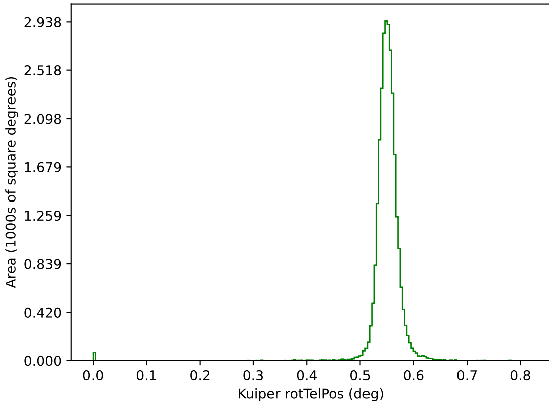
ddf_acor_sf10_ls15_lsr10_v3.4_10yrs g: Kuiper rotTelPos
