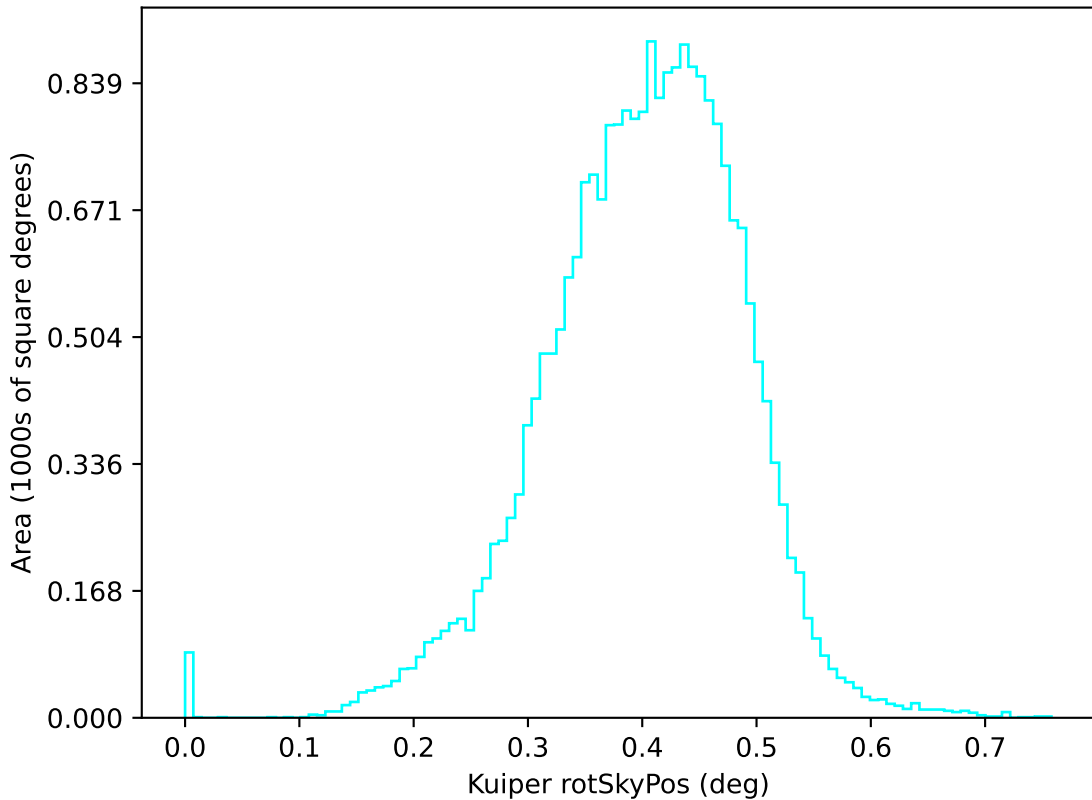
ddf_acor_sf10_lsf15_lsr10_v3.4_10yrs u: Kuiper rotSkyPos
