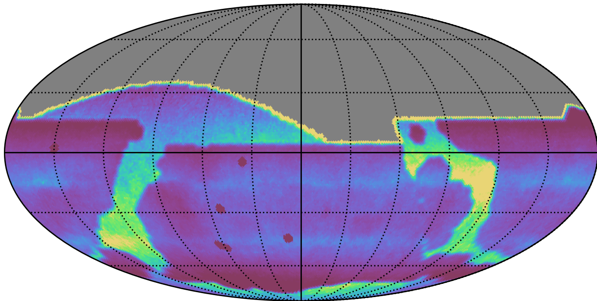
ddf_acor_sf10_lsf15_lsr10_v3.4_10yrs : DCRprecision
