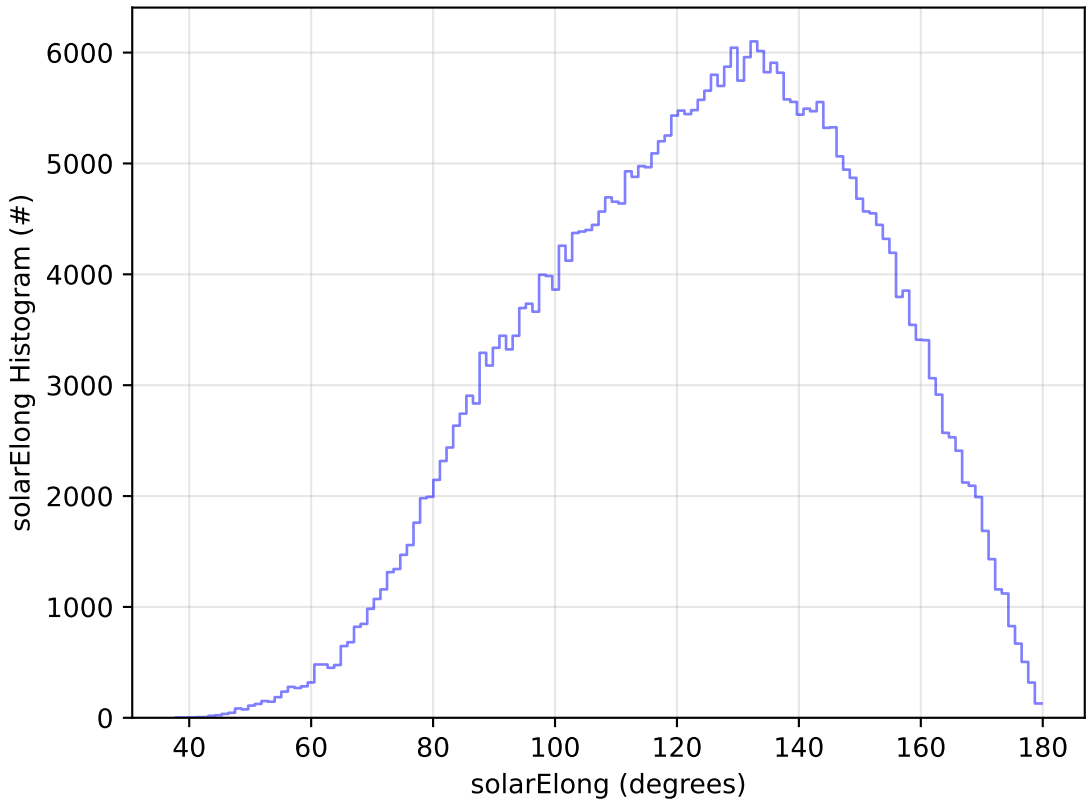
ddf_acor_sf10_lsf15_lsr10_v3.4_10yrs All sky y band: solarElong Histogram
