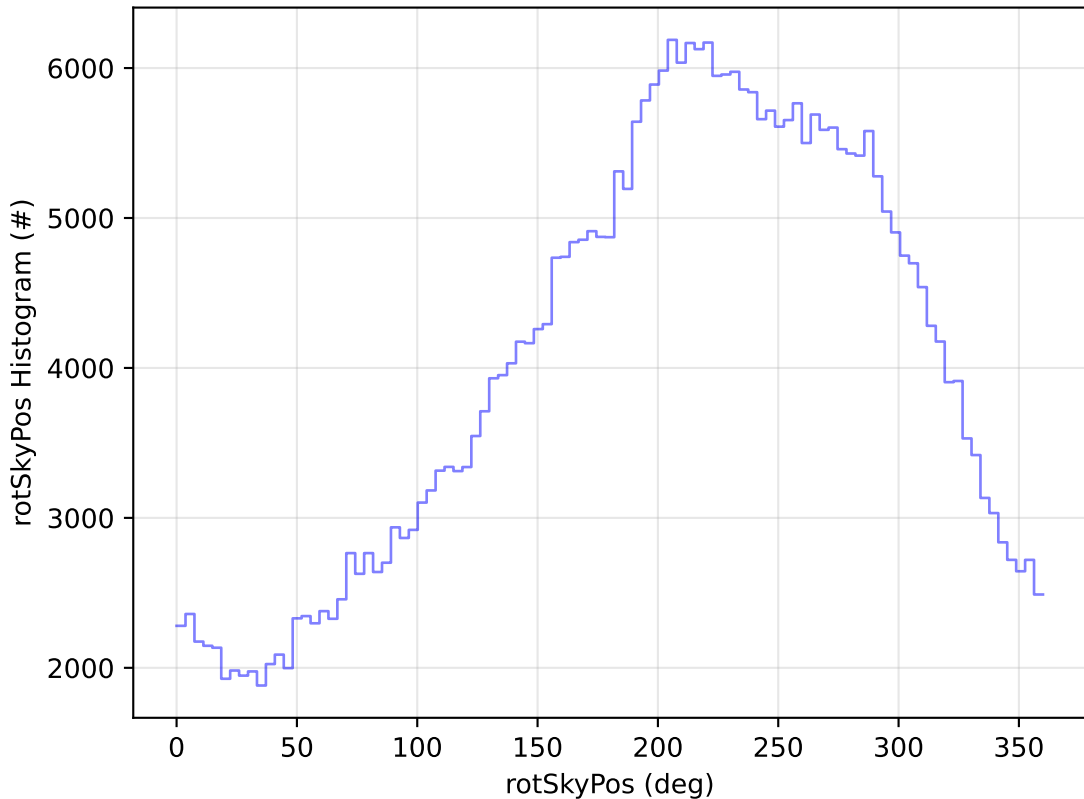
ddf_acor_sf10_lsf15_lsr10_v3.4_10yrs All sky y band: rotSkyPos Histogram
