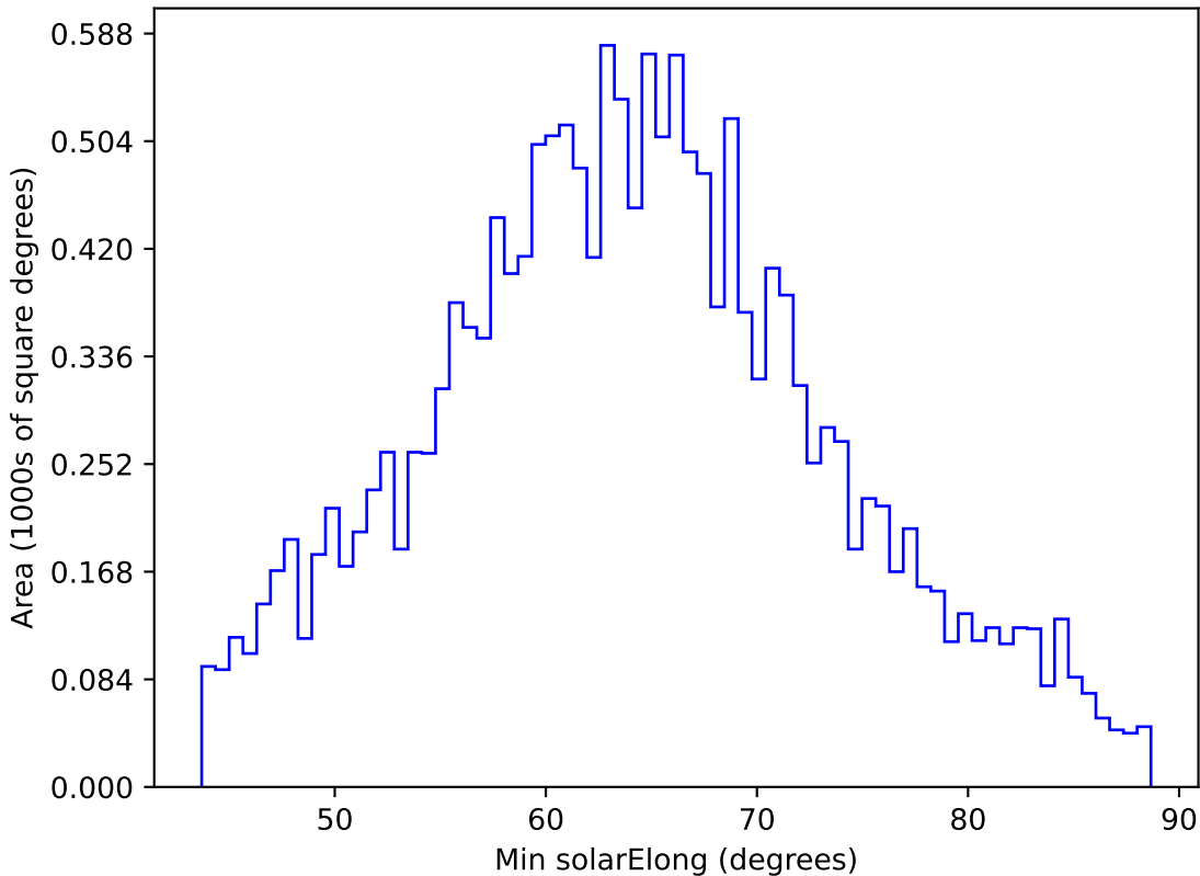
ddf_acor_sf10_lsf15_lsr10_v3.4_10yrs WFD y band: Min solarElong
